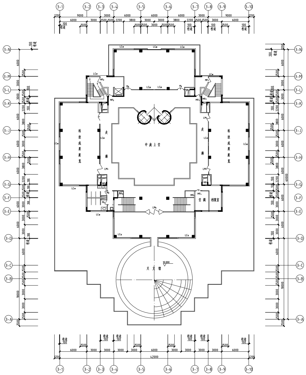
三层平面布置图
